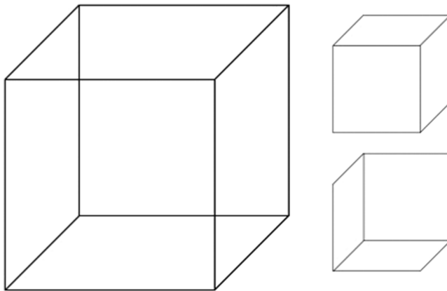
Der Necker-Würfel
