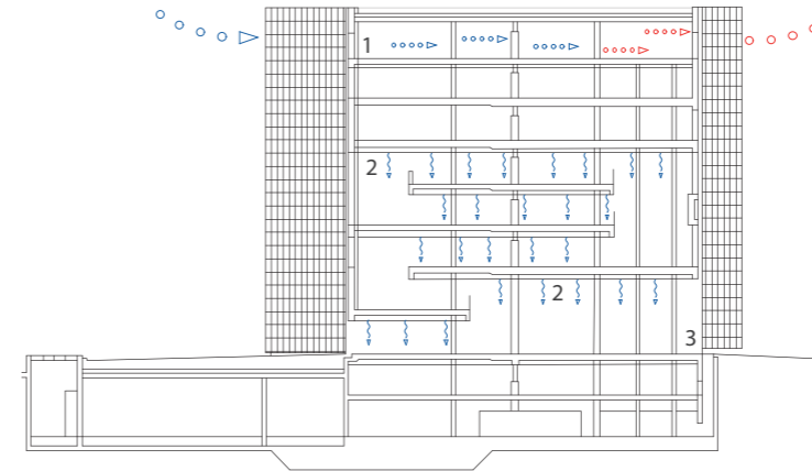
Schemaschnitt
