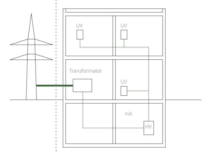
Stromversorgung größeres Nichtwohngebäude
