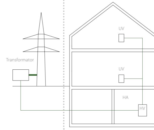
Stromversorgung Wohngebäude
