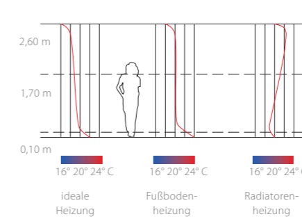
Temperaturschichtung im Aufenthaltsbereich des Menschen
