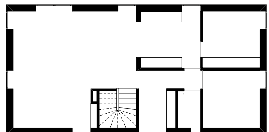
Grundriss Erdgeschoss
